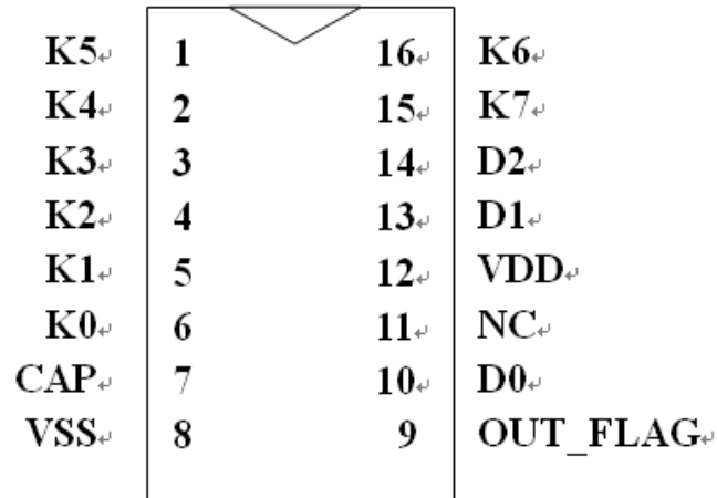
TTP272-AOBN ↙ 16-SOP-A ↙
