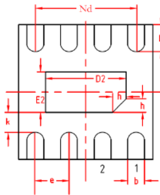
BOTTOM VIEW 背视图
