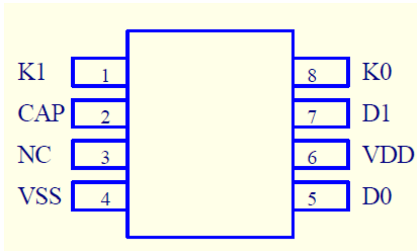
TTP277-AO8N 8-SOP-A
