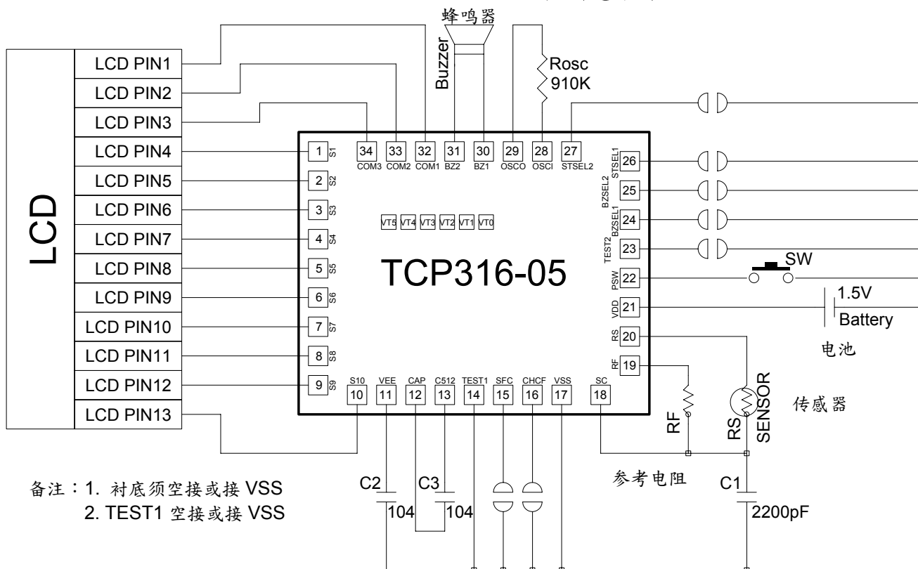
TCP316-05A/TCP316-05B 应用电路图
