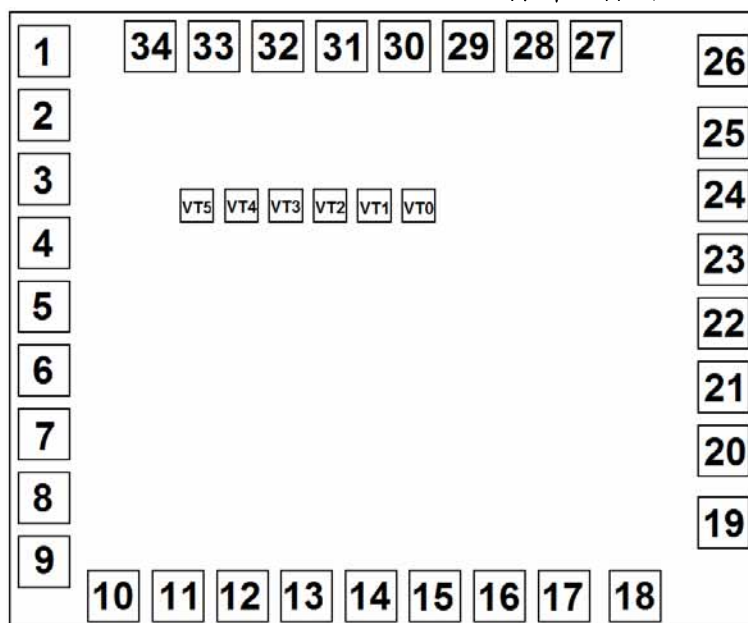
TCP316-05A/TCP316-05B 引脚坐标图
