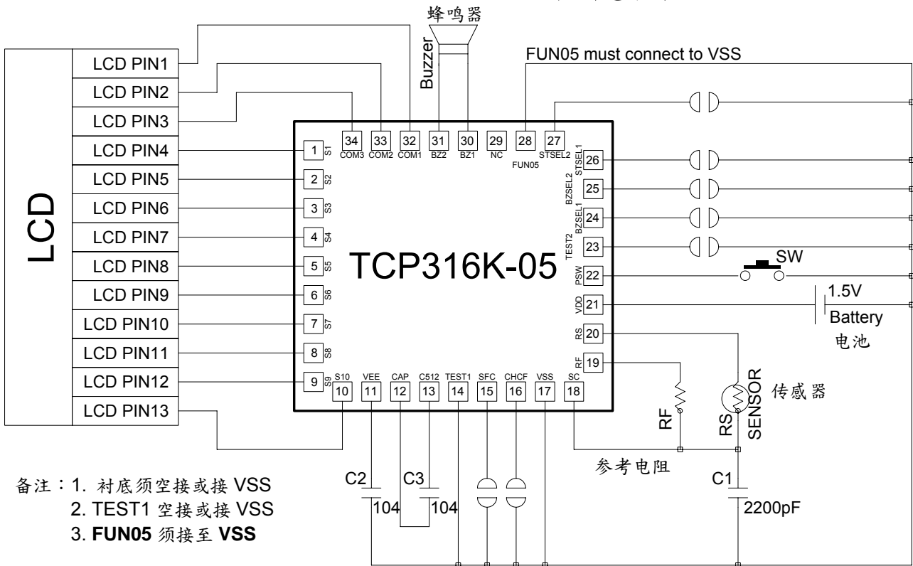
TCP316K-05A/TCP316K-05B 应用电路图
