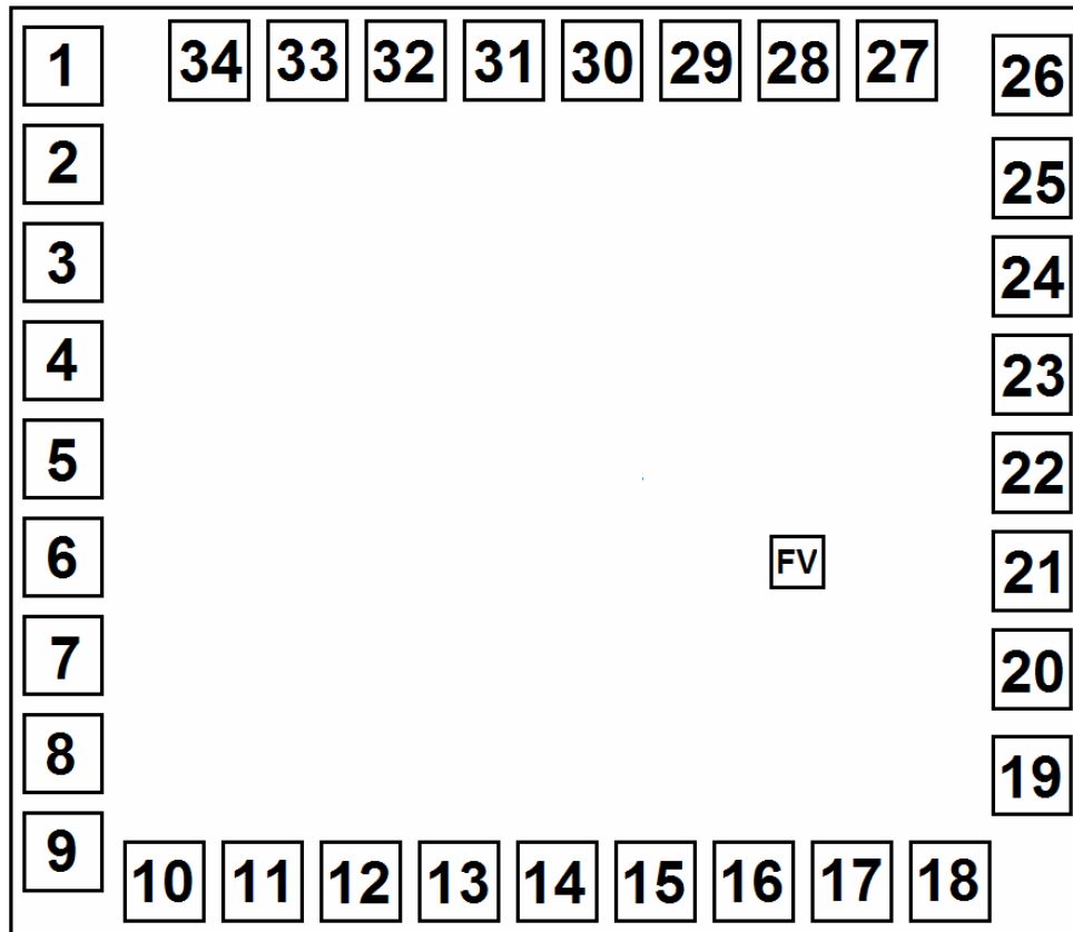
TCP316K-05A/TCP316K-05B 引脚坐标图
