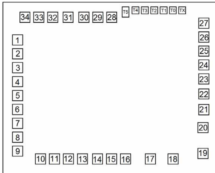
TCP310A/TCP310B 引脚坐标图
