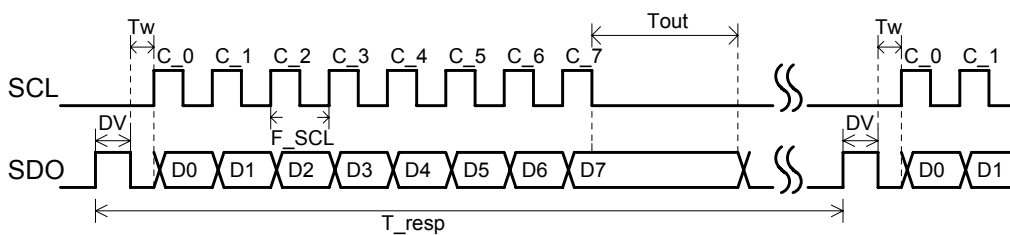
图3-4-3: 8键输入, 高电平有效时序
