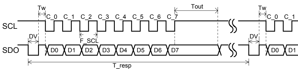
图3-4-4: 8输入键, 低电平有效时序
